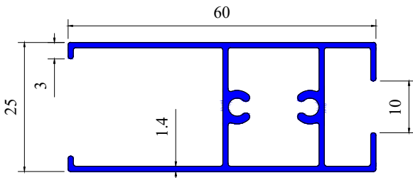
SHUTTER TOP&BOTTOMSID
